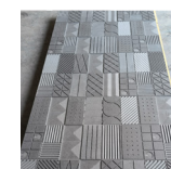
SN-S拉槽款-28号组合拼花 Number 28 parquet 规格SIZE1220*2440*12
